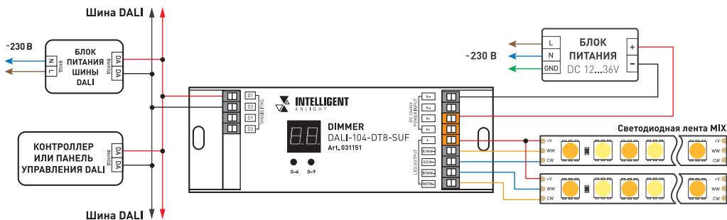
Рисунок 3. Пример схемы подключения диммера DALI-014-DT8-SUF в режиме Tc (управление светодиодными лентами MIX)
